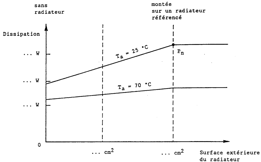
Figure 1: Courbe de réduction de la dissipation en fonction de la surface du radiateur
